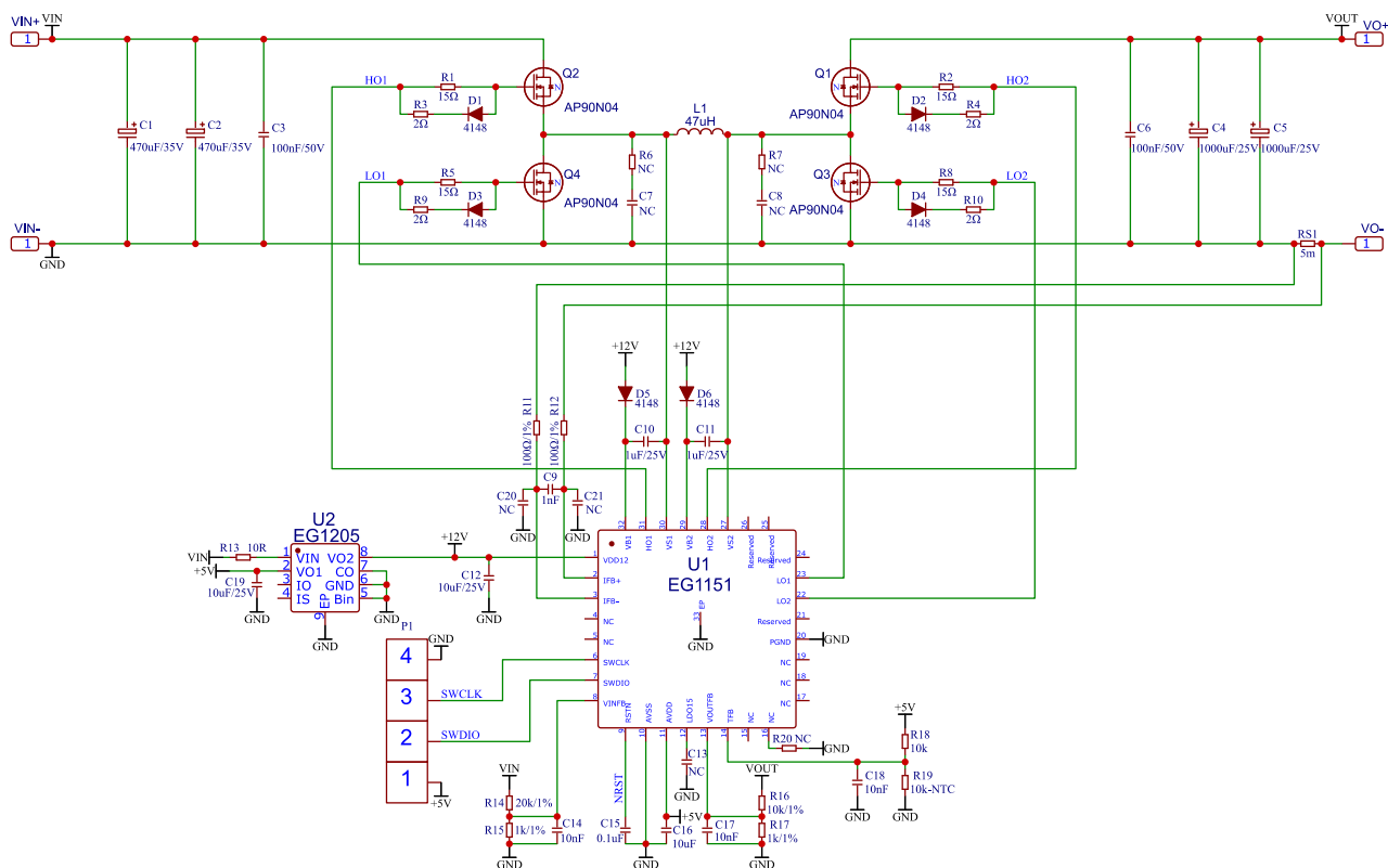
图 6-1. EG1151-15V10A 恒压恒流方案典型应用电路图
