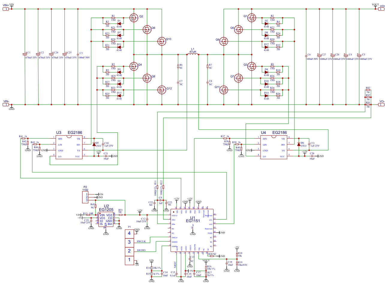
图 6-2. EG1151-15V50A 恒压恒流大功率扩流方案典型应用电路图
